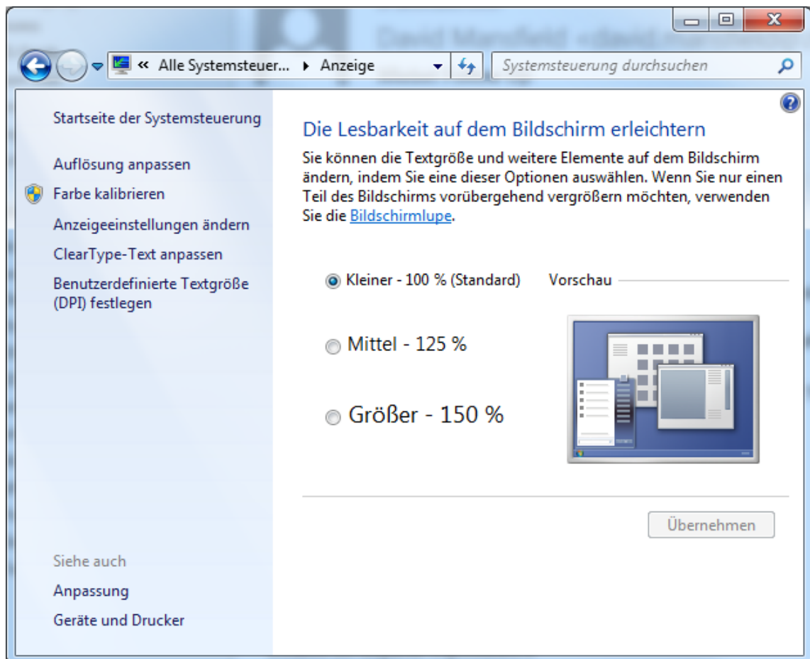
Abb. 3: Windows Schriftgrößeneinstellung
