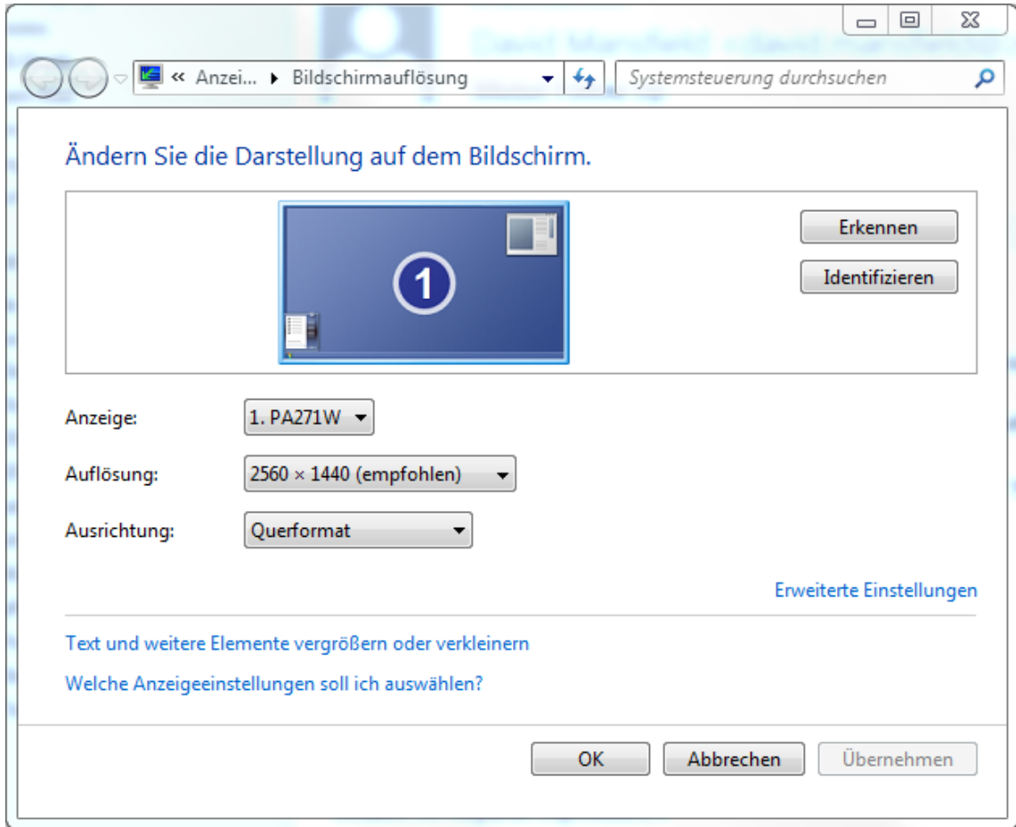
Abb. 2: Windows-Dialog Bildschirmauflösung
